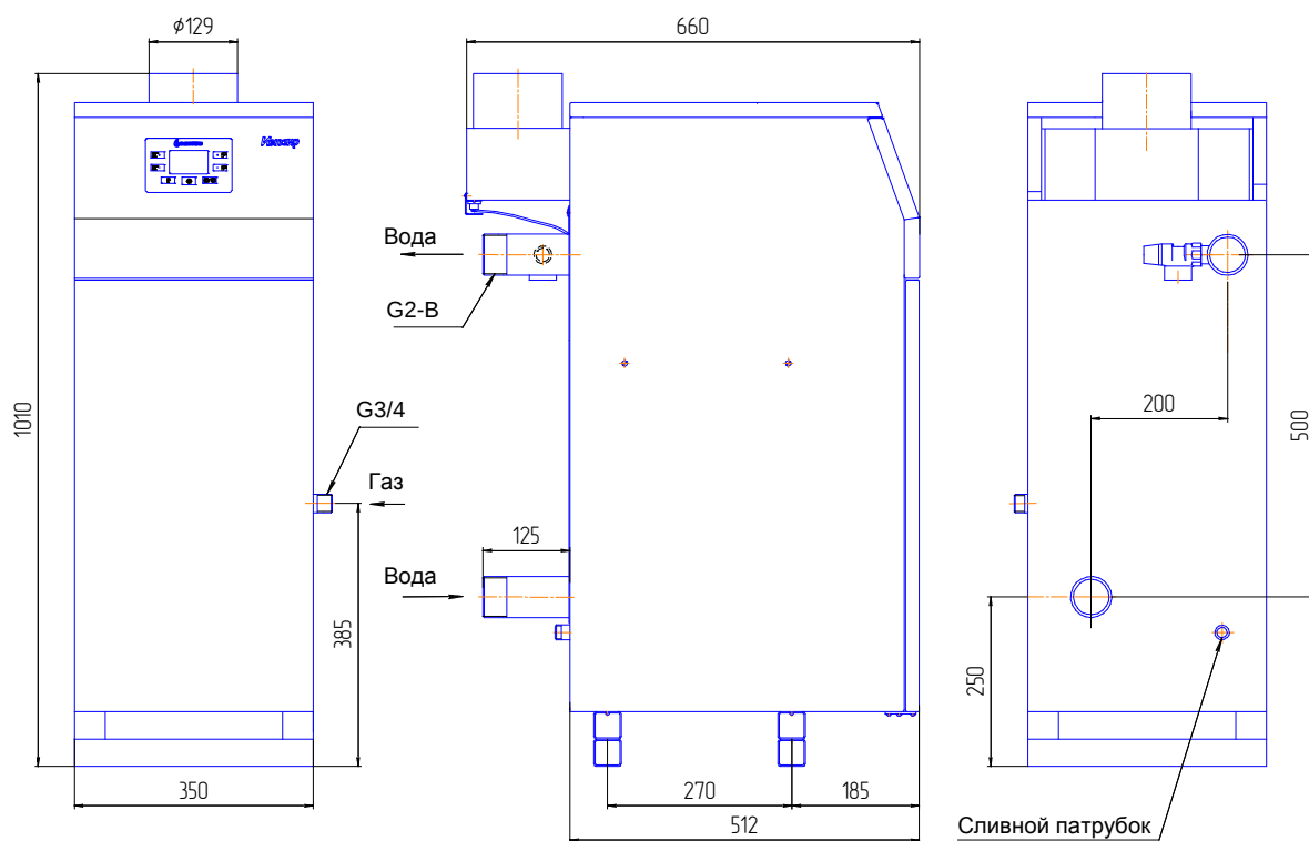
Рисунок 3. Габаритные и присоединительные размеры котлов.
